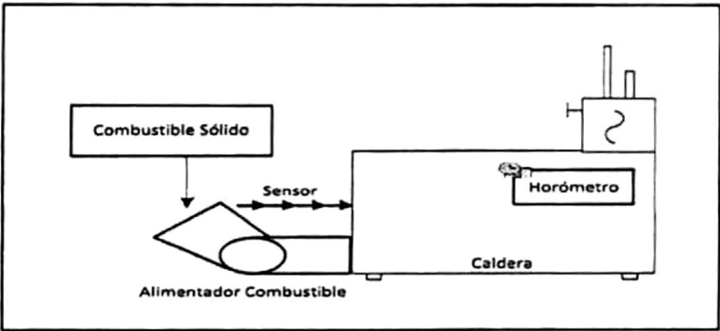
Figura 2 - Caldera con combustible sólido
